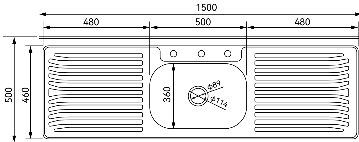
正视图 / Front View
