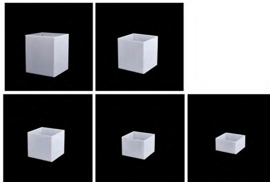
亚克力五面方柱 1037W 规格/Size ① 180×180×100mm ② 200×200×150mm ③ 220×220×200mm ④ 240×240×250mm ⑤ 260×260×300mm
