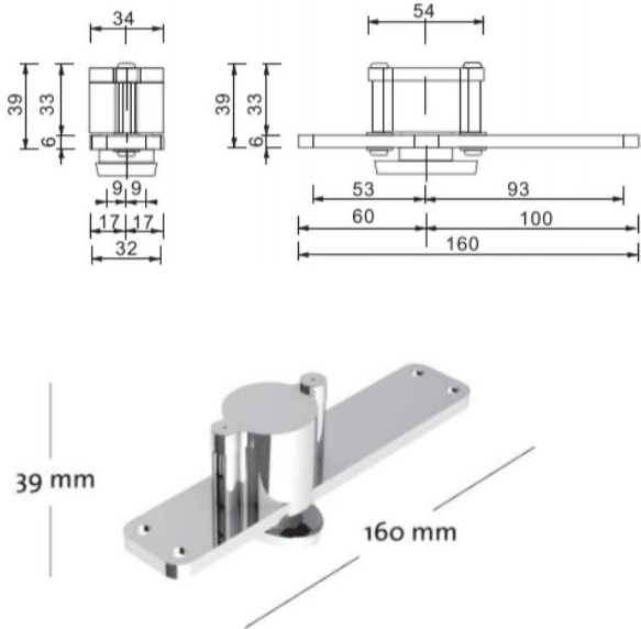
产品尺寸
