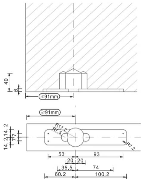
开槽图纸
