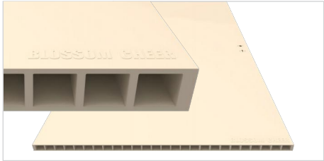
Standard pure WPC structure* 标准纯 WPC 结构 *
