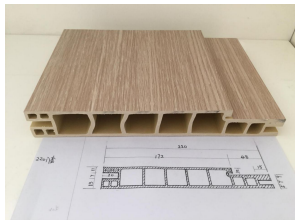
22031 Frame
