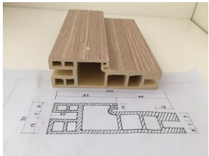
10031 Frame
