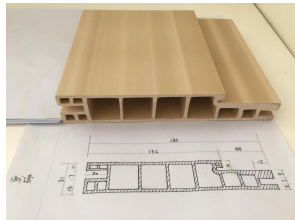
18031 Frame
