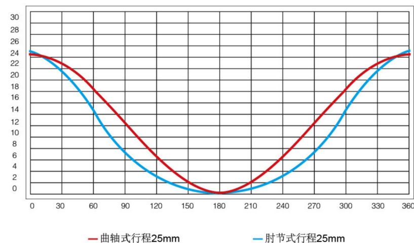
肘节连杆结构与曲轴结构冲压曲线对比图
