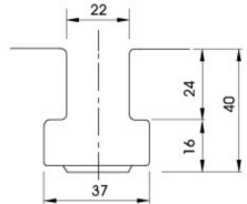
T型沟 II 型
