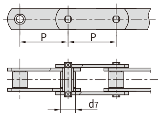
2.带S型小滚子 2.with S small rollers type
