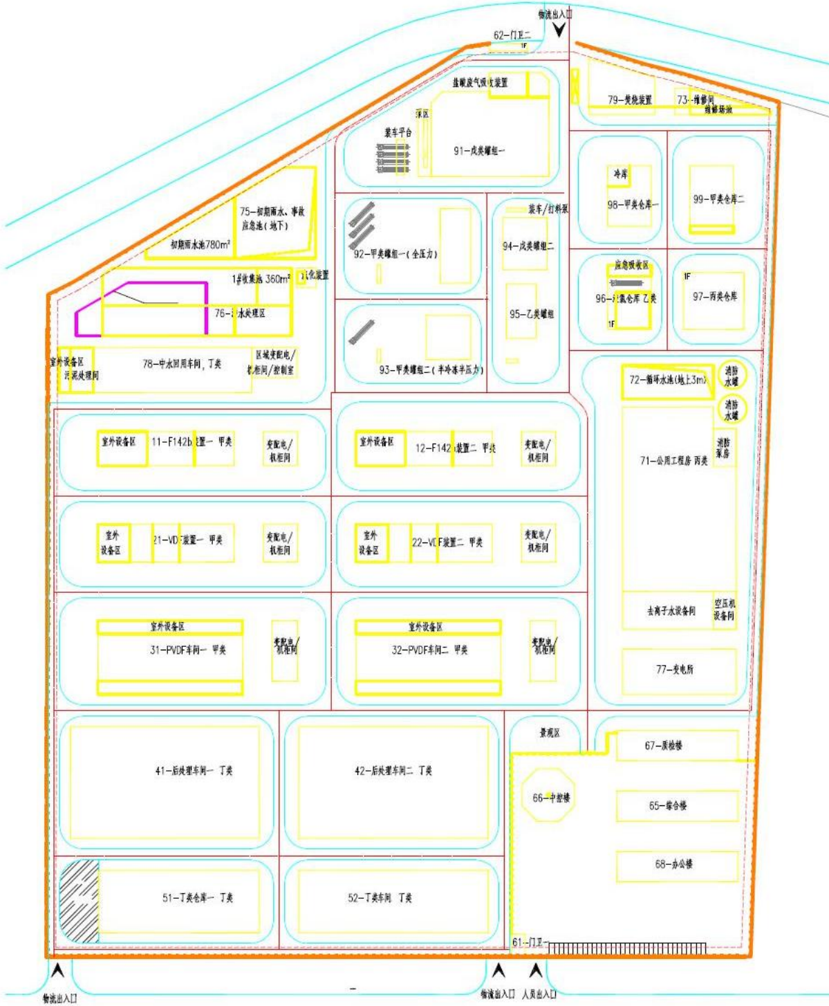
图 3-1 全厂平面布置图
