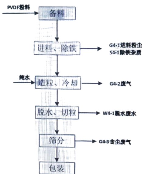
图 3-5 偏氟乙烯聚合物造粒车间工艺流程及产污节点图
