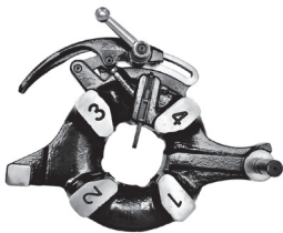
443 die head
