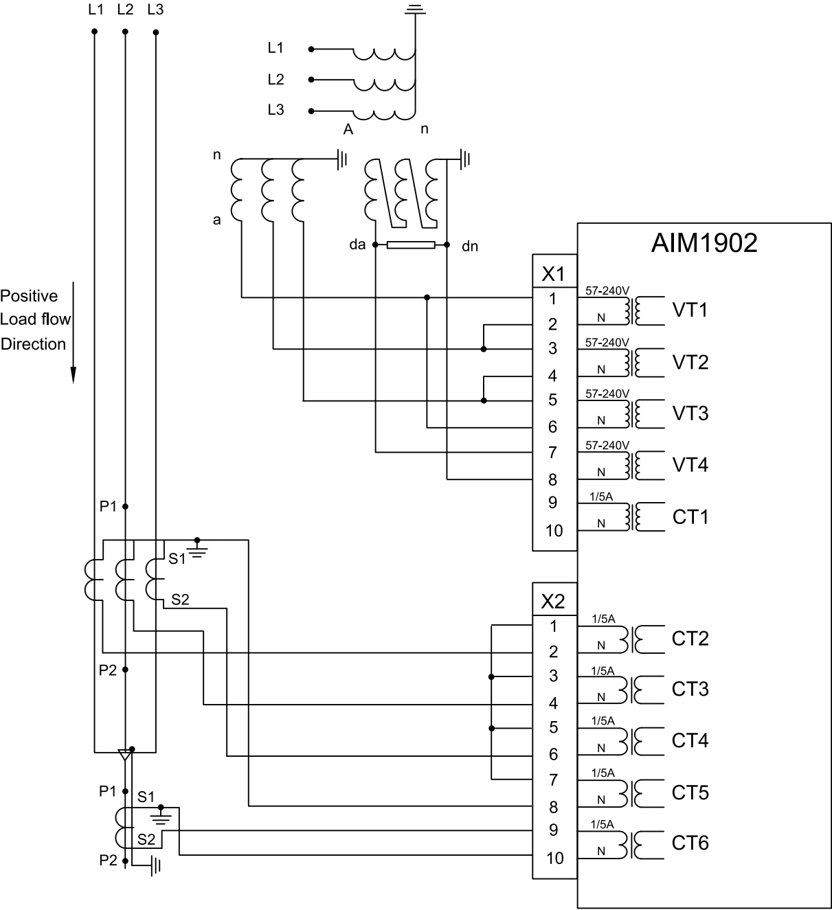
Figure 33: AIM1902 module
