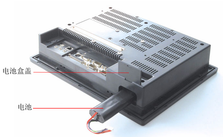
图 2.4: PPC-L128T 底视图
