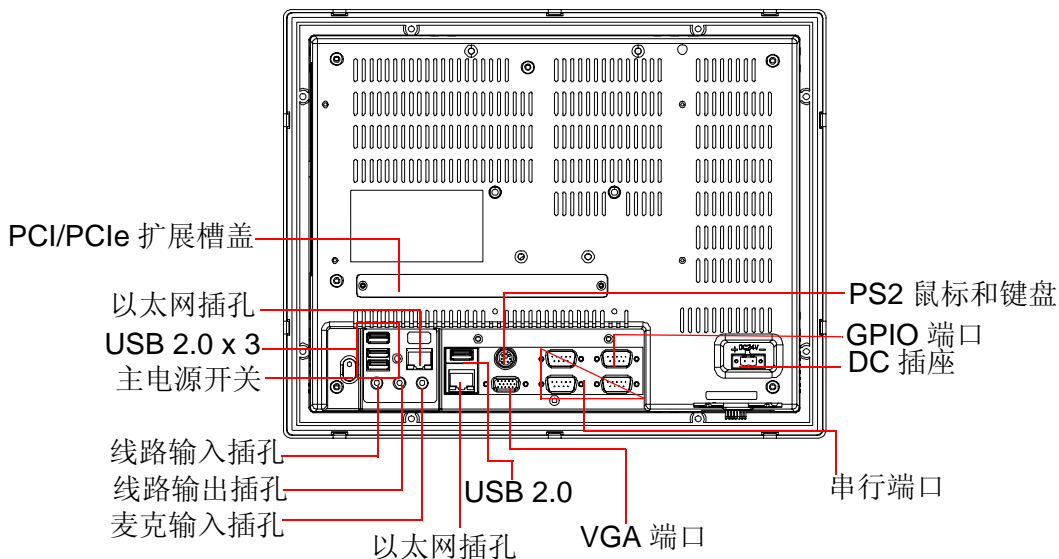
图 2.2: PPC-L128T 后视图
