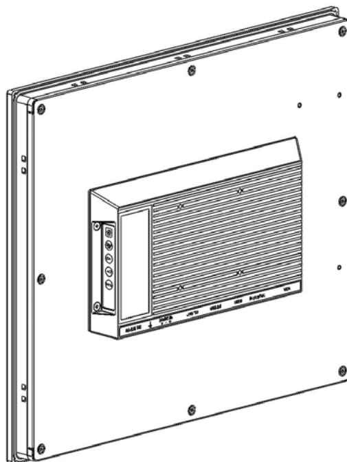
圖 2.4 VESA 安裝
