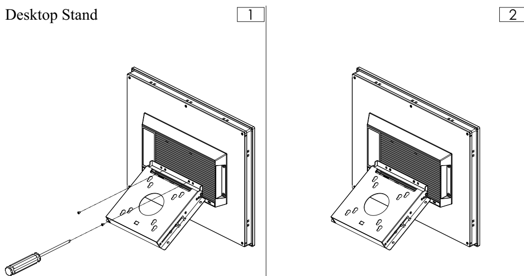
圖 2.3 桌面安裝
