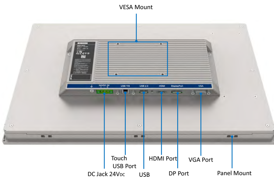
圖 1.2 FPM-715W - I/O Port Arrangement
