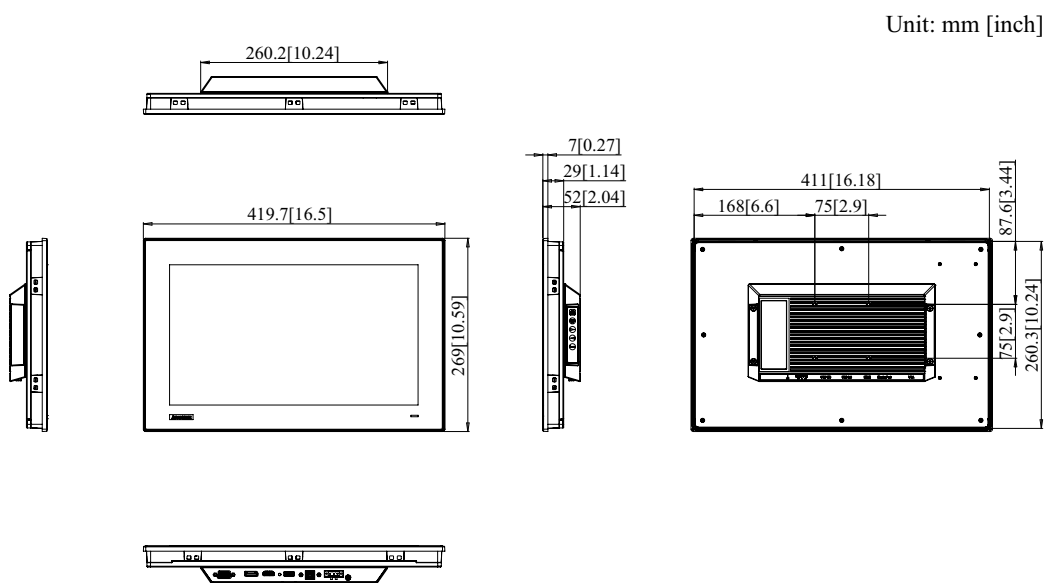
圖 1.3 FPM-715/717/719 尺寸
