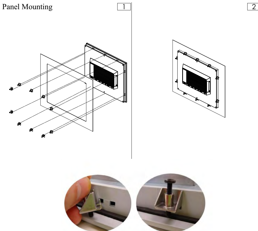
圖 2.1 面板式安裝
