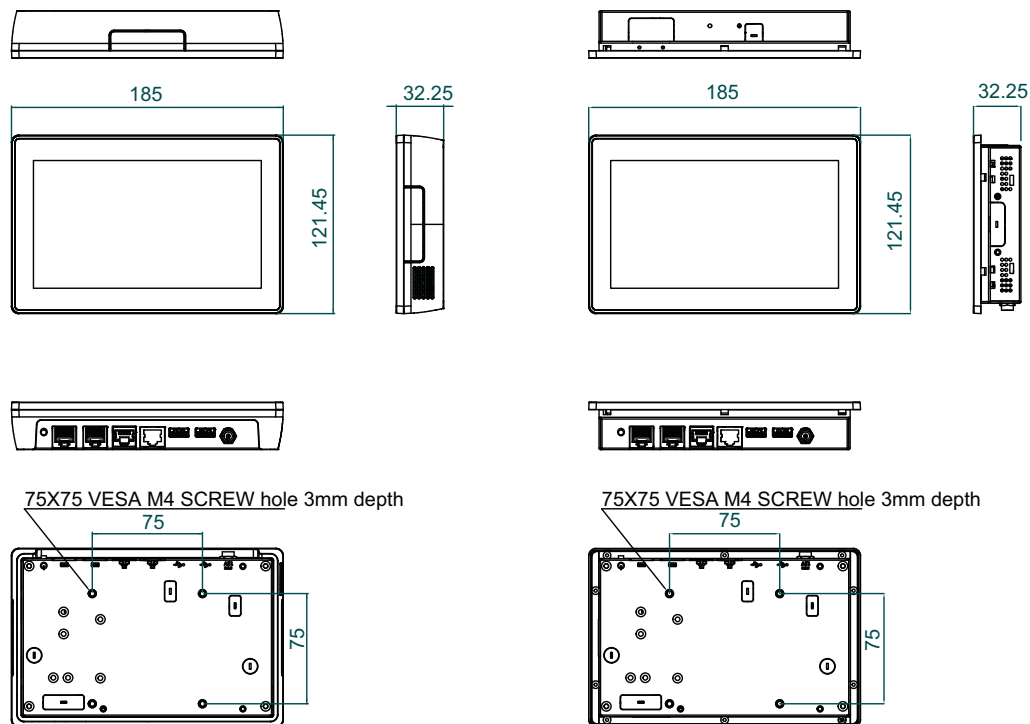
圖 1.1：UTC-307 尺寸圖
