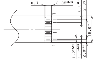
コネクタ接続部 (導通面)
