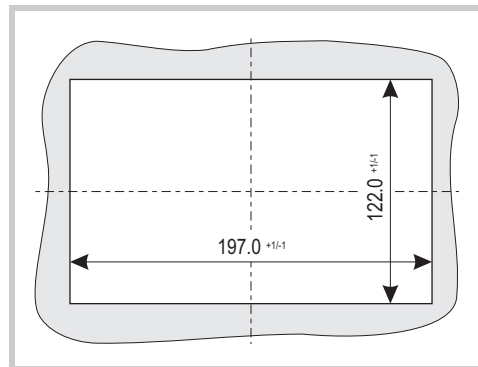
Abb. 30 Einbuausschnitt für 7,0"-Geräte
