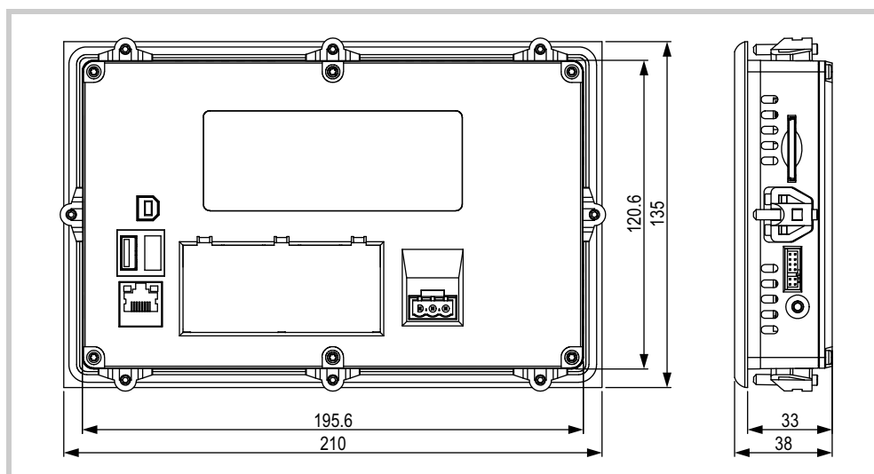
Abb. 42 Mechanische Abmessungen der 7,0"-Geräte in mm
