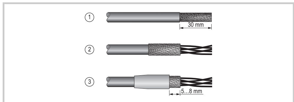
Abb. 9 Kabelschirm anschliessen
