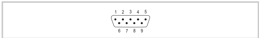
Abb. 26 RS485-Schnittstelle (9-polig, D-Sub, male, UNC)
