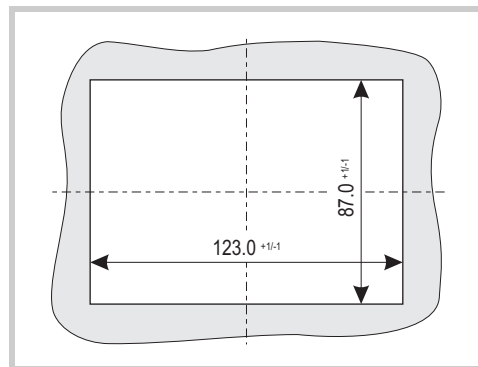
Abb. 28 Einbuausschnitt für 3,5"-Geräte
