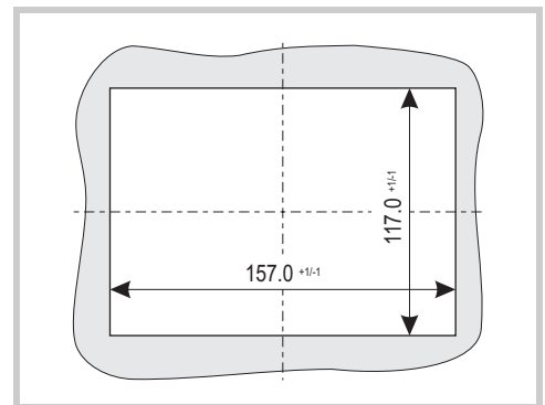
Abb. 29 Einbuausschnitt für 5,7"-Geräte
