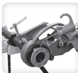
套丝操作
