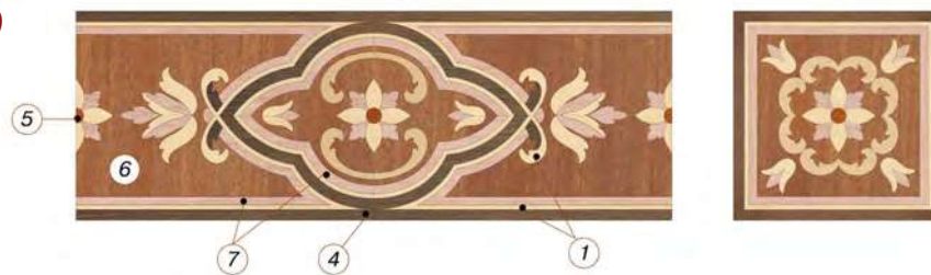
• Border "Maranta 1" (1912) width 300 mm
